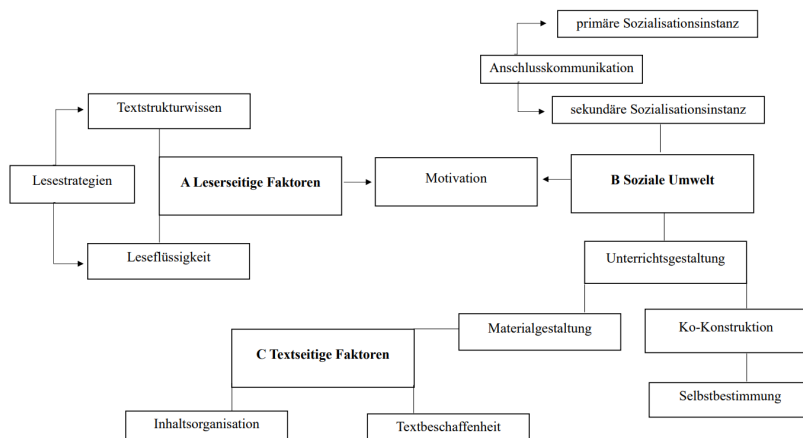
Abbildung 7: Multifaktorielles Lesekompetenzmodell
